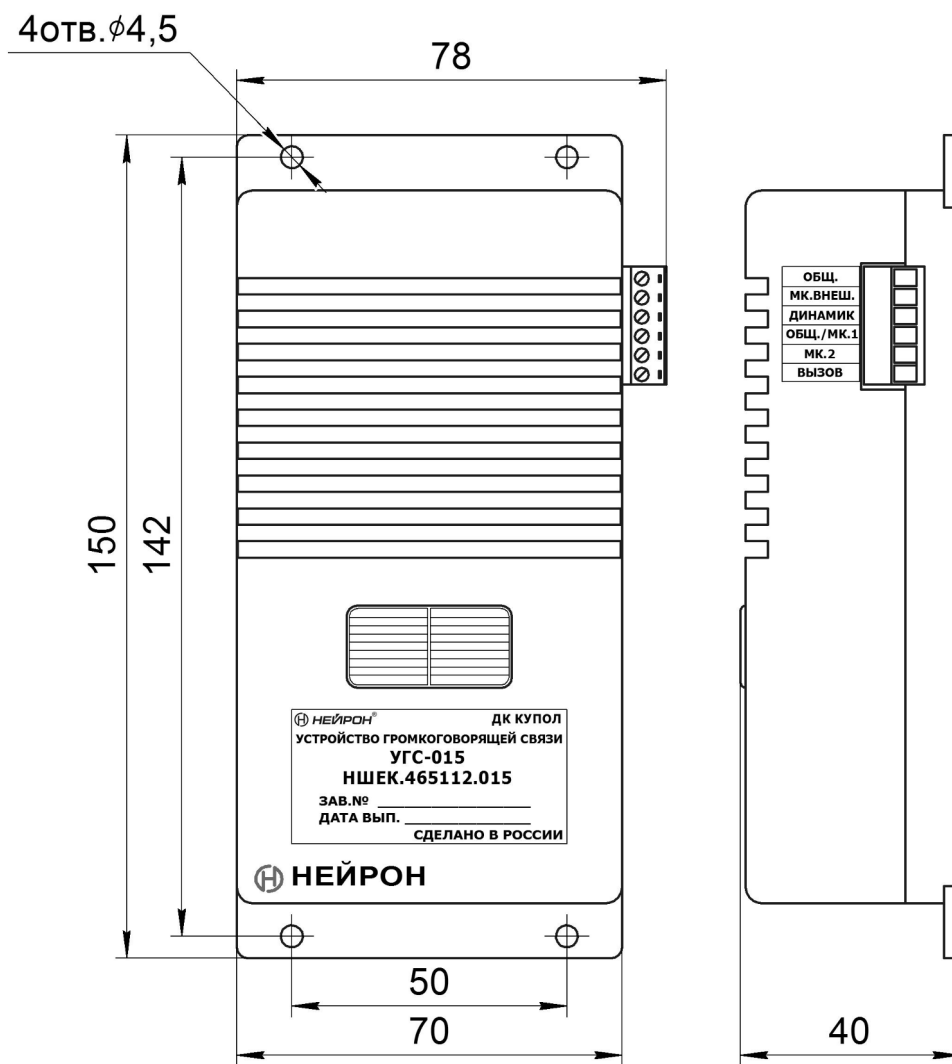
Рис.1 Внешний вид Устройства громкоговорящей связи УГС-015 НШЕК.465112.015
